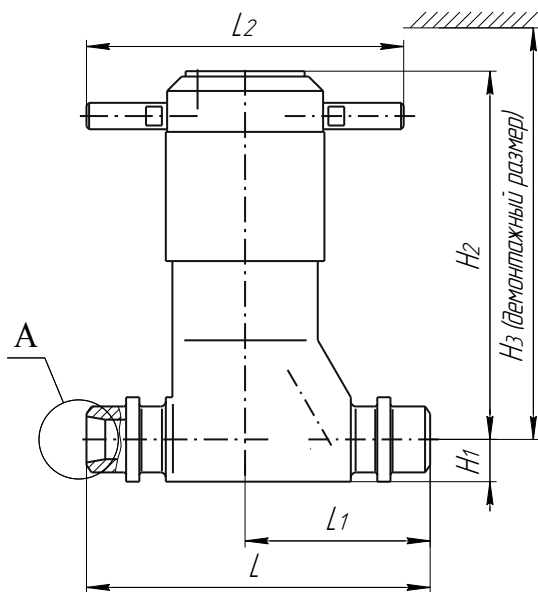
Рисунок 1 – DN 10, 15
