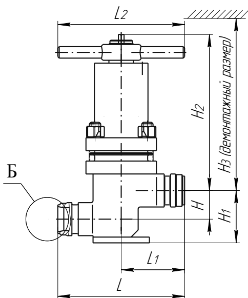
Рисунок 2 – DN 20, 32, 50
